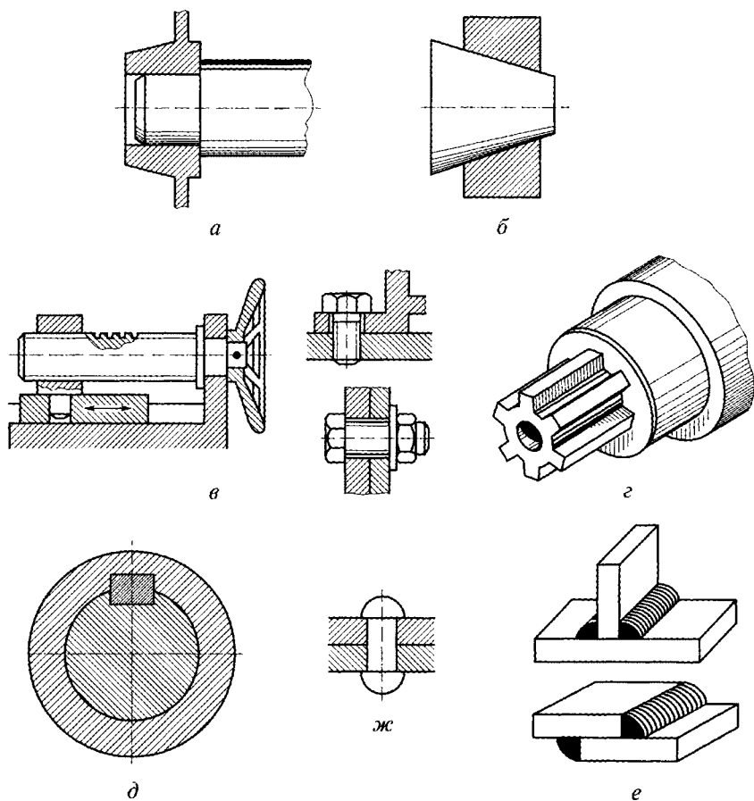
Рис. 2.7. Соединения поверхностей:
