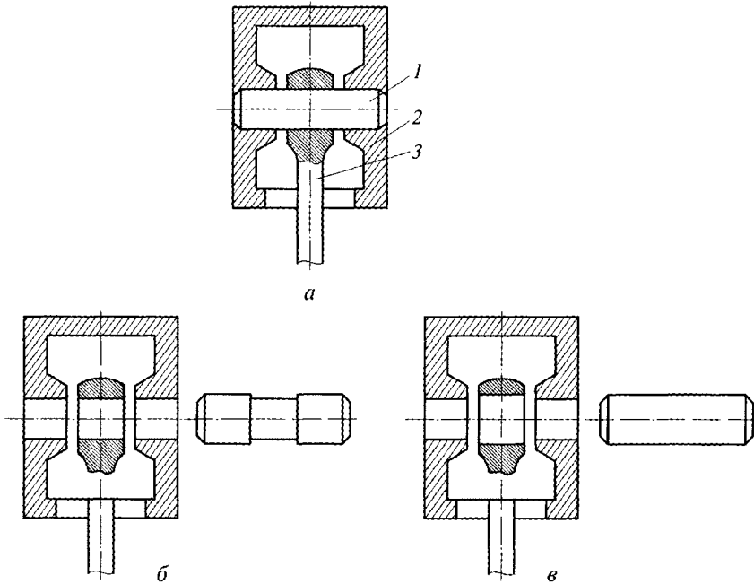
Рис. 2.13. Примеры соединений ( а—в ): 1 — поршневой палец; 2 — поршень; 3 — шатун
