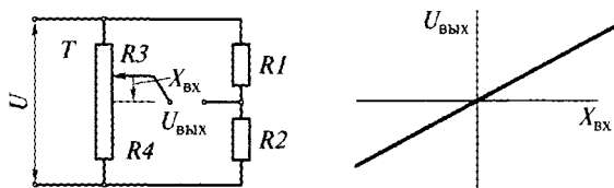
Рис. 1.11. Мостовая схема потенциометрического датчика и его характеристика
