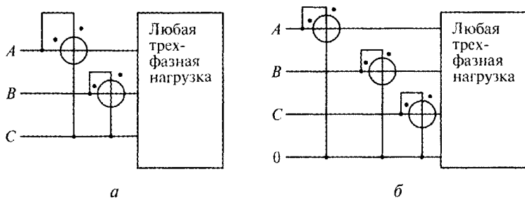
Рис. 1.37. Схемы измерения мощности на переменном токе:
