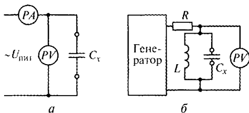
Рис. 1.35. Схемы измерения емкости:
