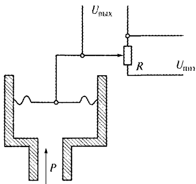
Рис. 1.17. Датчик давления
