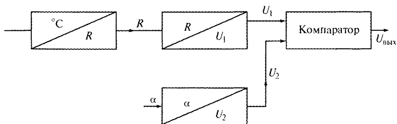
Рис. 1.20. Блок-схема термореле
