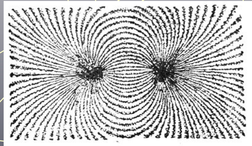
Магнитное поле разноименных
